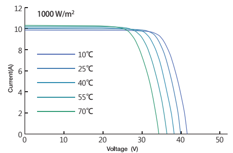
不同工作温度下电流电压曲线图
